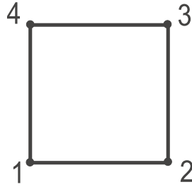
Abbildung 3.5: Quadrat mit Nummerierung
