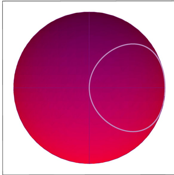
Abbildung 4.9: Projektive Parabel auf der Einheitsscheibe.
