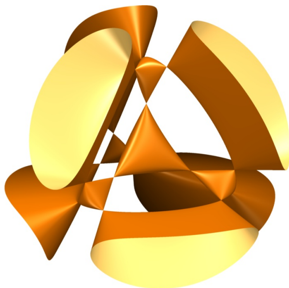
Abbildung 1.8: Kummerquartik
