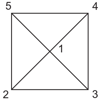
Abbildung 3.3: Quadrat im Oktaeder
