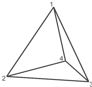
Abbildung 3.6: Tetraeder mit Nummerierung
