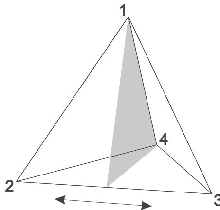
Abbildung 1.3: Spiegelsymmetrie (2,3) des Tetraeders
