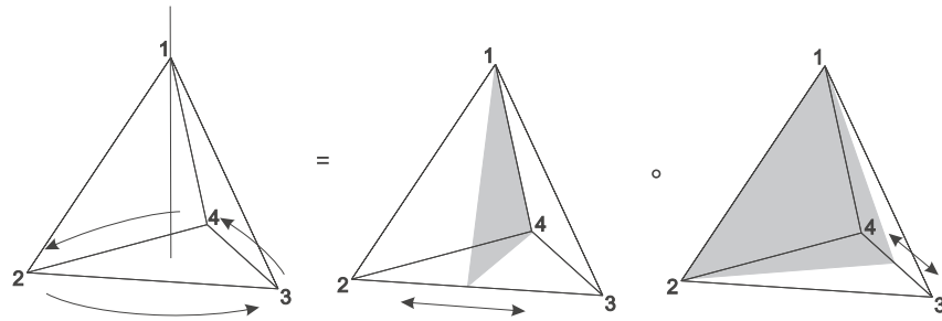
Abbildung 1.2: Komposition von zwei Symmetrien des Tetraeders
