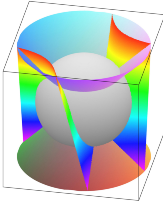
Abbildung 4.15: Durchschnitt von drei Kegelschnitten
