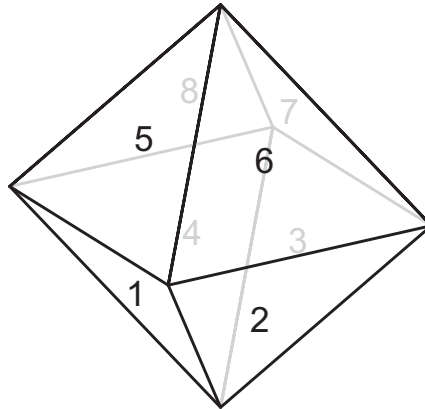
Abbildung 3.7: Oktaeder mit Seitennummerierung
