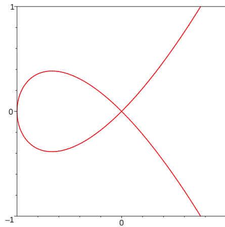
Abbildung 4.14: Nodale Kubik
