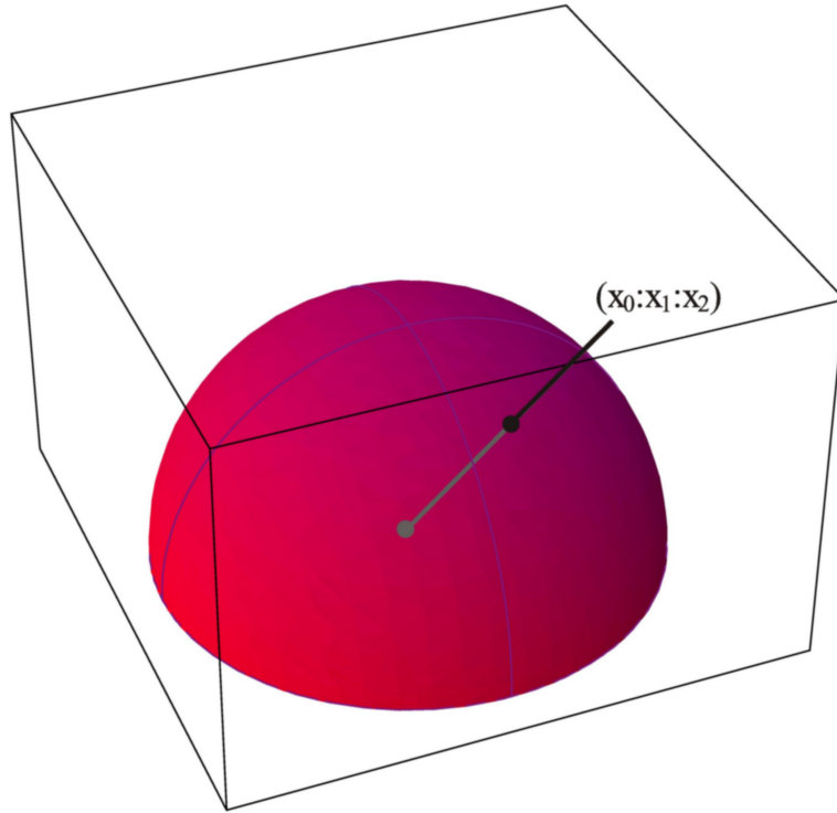
Abbildung 4.6: Projektiver Raum \mathbb{P}^2(\mathbb{R}) .
