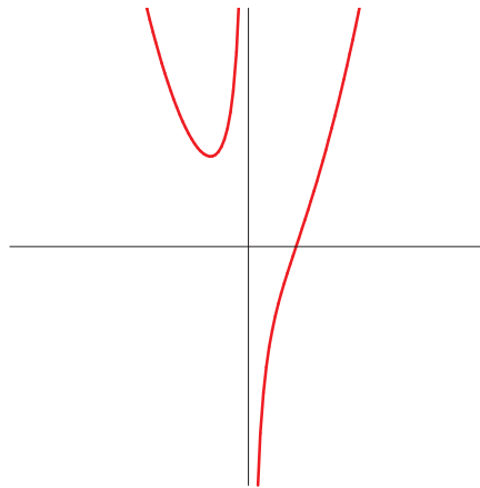
Abbildung 4.1: Graph einer rationalen Funktion
