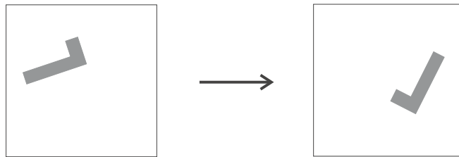
Abbildung 3.2: Beispiel einer Bewegung des \mathbb{R}^2 .
