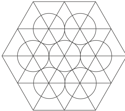
Abbildung 6.1: Hexagonale Kugelpackung
