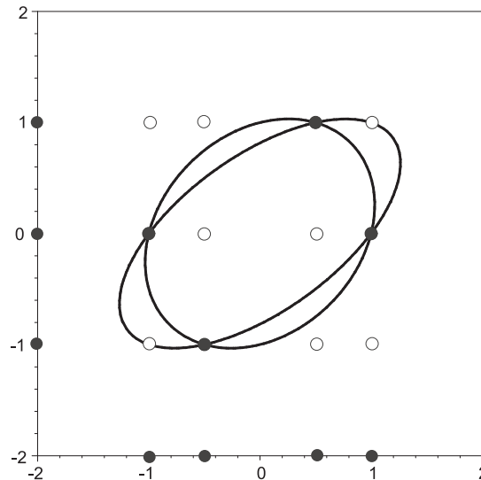
Abbildung 4.2: Projektionen des Durchschnitts von zwei Ellipsen
