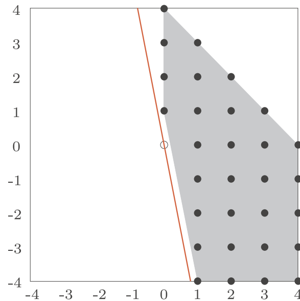
Abbildung 4.13: M_{\succ} für die Ordnung lp und Monome vom Grad \leq 4
