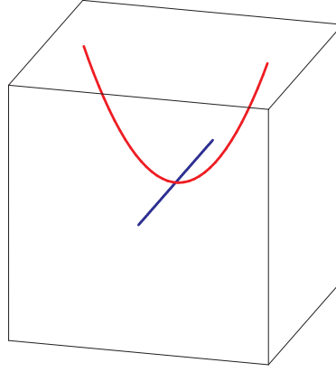
Abbildung 4.11: Vereinigung von algebraischen Mengen
