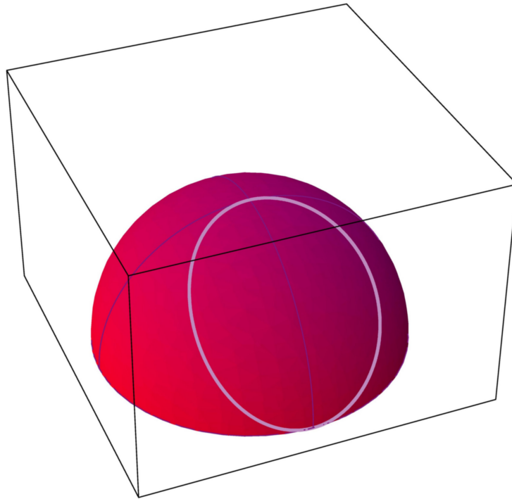
Abbildung 4.8: Projektive Parabel
