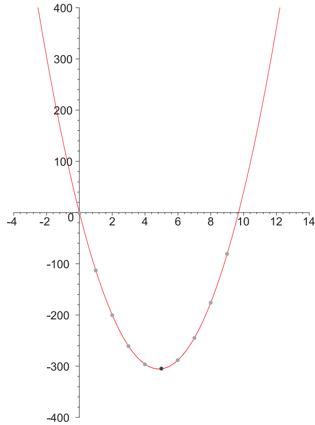
Abbildung 6.3: Längendifferenz vor Reduktion
