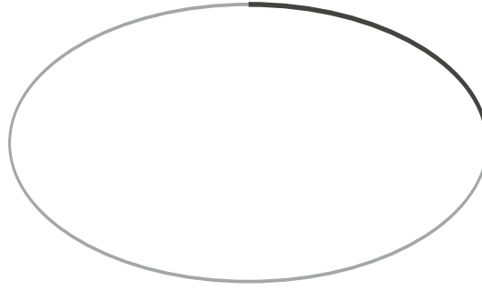
Abbildung 4.3: Ellipsenabschnitt
