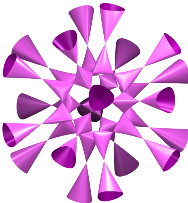
Abbildung 1.10: Barthsextik
