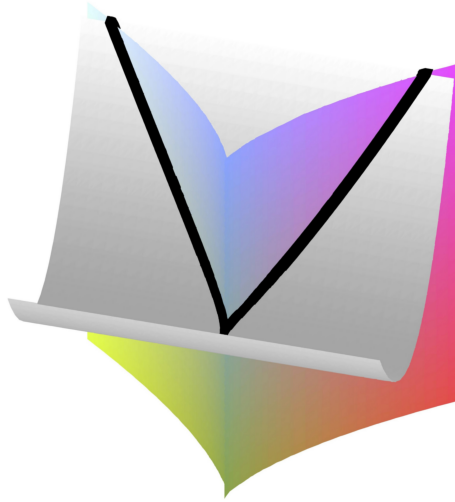
Abbildung 4.10: Kurve gegeben durch eine Parametrisierung bzw. implizite Gleichungen
