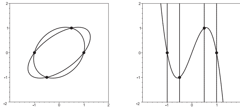
Abbildung 1.7: Buchberger-Algorithmus für den Schnitt von zwei Ellipsen
