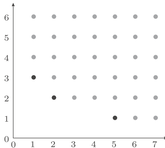
Abbildung 4.5: Monome in \langle xy^3, x^2y^2, x^5y \rangle
