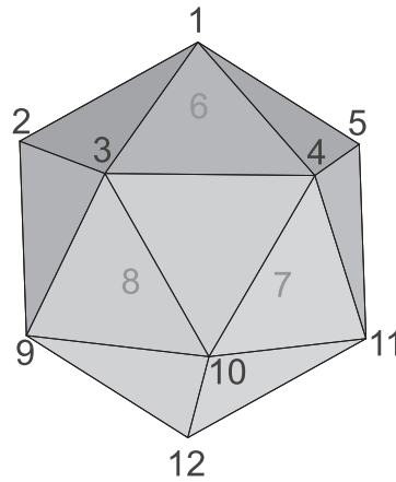
Abbildung 3.9: Ikosaeder mit Nummerierung
