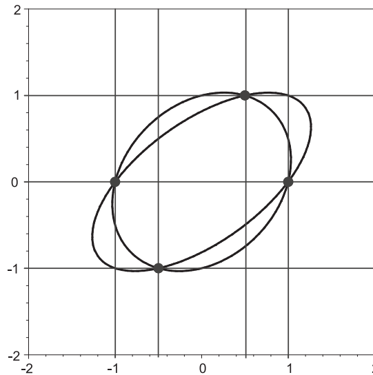
Abbildung 4.4: Elimination für den Durchschnitt von zwei Ellipsen
