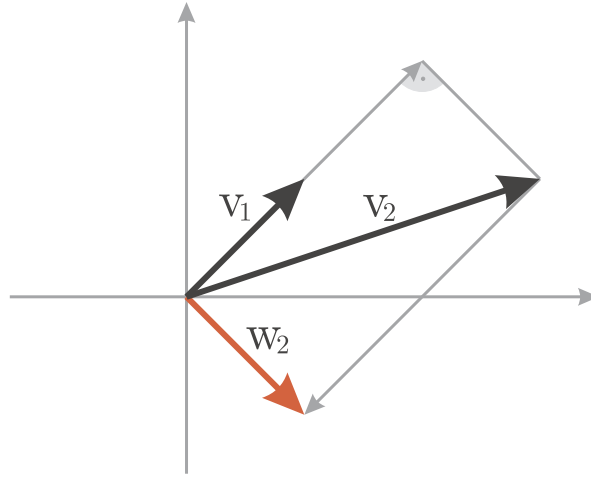
Abbildung 6.2: Gram-Schmidt-Verfahren und Projektion
