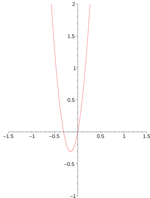
Abbildung 6.4: Längendifferenz nach Reduktion
