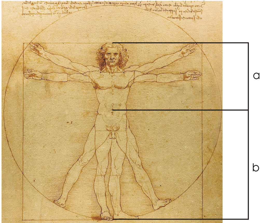
Abbildung 6.6: Proportionen des Menschen von Leonardo da Vinci
