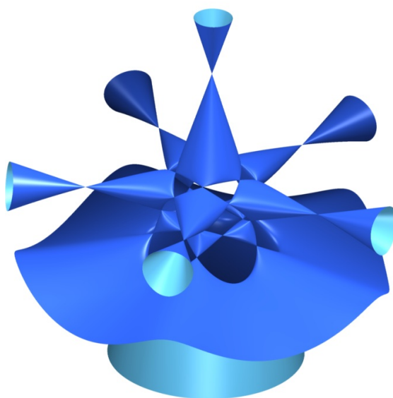
Abbildung 1.9: Togliattiquintik
