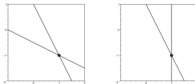
Abbildung 1.6: Gauß-Elimination für den Durchschnitt von zwei Geraden
