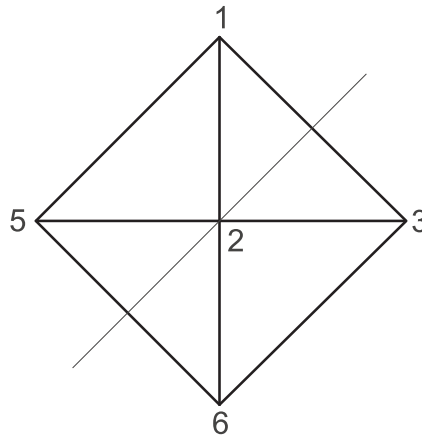
Abbildung 3.4: Spiegelung (1, 3)(5, 6) als Symmetrie des Oktaeders
