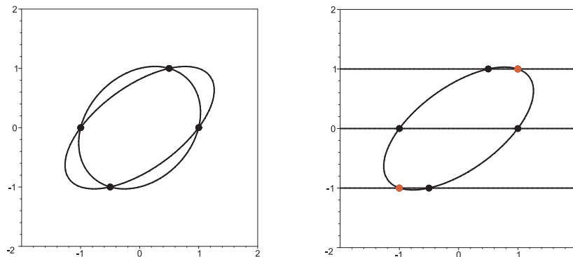
Abbildung 4.12: Buchberger-Algorithmus mit x > y für den Schnitt von zwei Ellipsen
