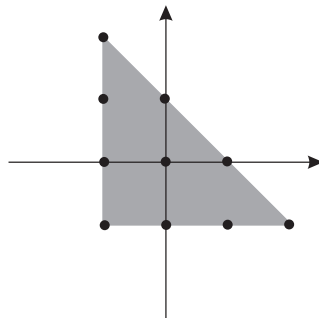
Abbildung 1.5: Polyeder
