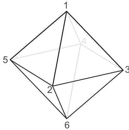
Abbildung 3.1: Oktaeder
