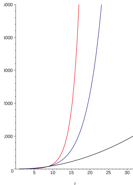
Abbildung 2.1: Laufzeitvergleich zwischen Multiplikation, quadratischem Sieb und Probedivision
