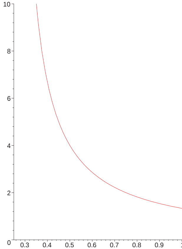
Abbildung 6.5: Skalierungsfaktor \tau in Abhängigkeit von \delta .
