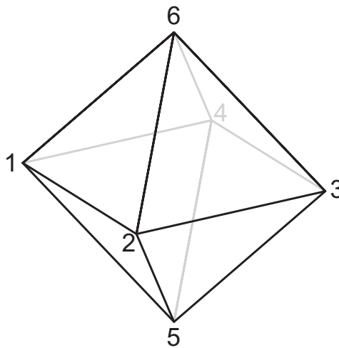
Abbildung 3.8: Oktaeder mit Eckennummerierung
